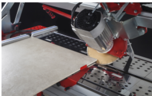
Taiere la 45°
