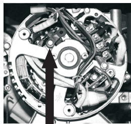
Рисунок D - Видте местоположение на въглеродните четки. Този елемент може евентуално да се наложи да бъде заменен, когато се износи.
