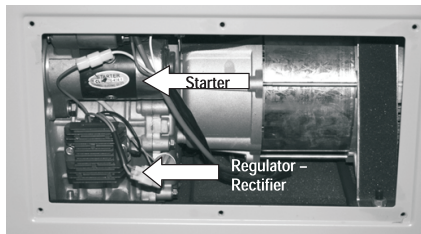
Рисунок С - Видте местоположението на задния панел за достъп, който е премахнат. Можете да видите местоположението на стартера и регулатора/изправителя за 12 В стартовата батерия. Стартерният двигател е разположен над регулатора/изправителя.
