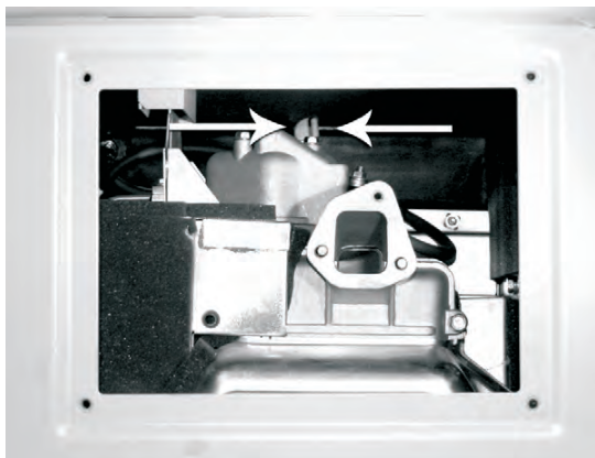
Рисунок А - Отстранете страничния панел, след това отстранете въздушния филтър. Намерете "Червения" лост за декомпресия (Снимката по-горе го показва в позиция НАГОРЕ). Натиснете лоста надолу - това ще държи изпускателния клапан отворен. Сменете въздушния филтър. Стартирайте двигателя. Ще забележите, че пружинният лост автоматично ще се върне в позиция НАГОРЕ (Също посочен като вал за декомпресия на диаграмата на
