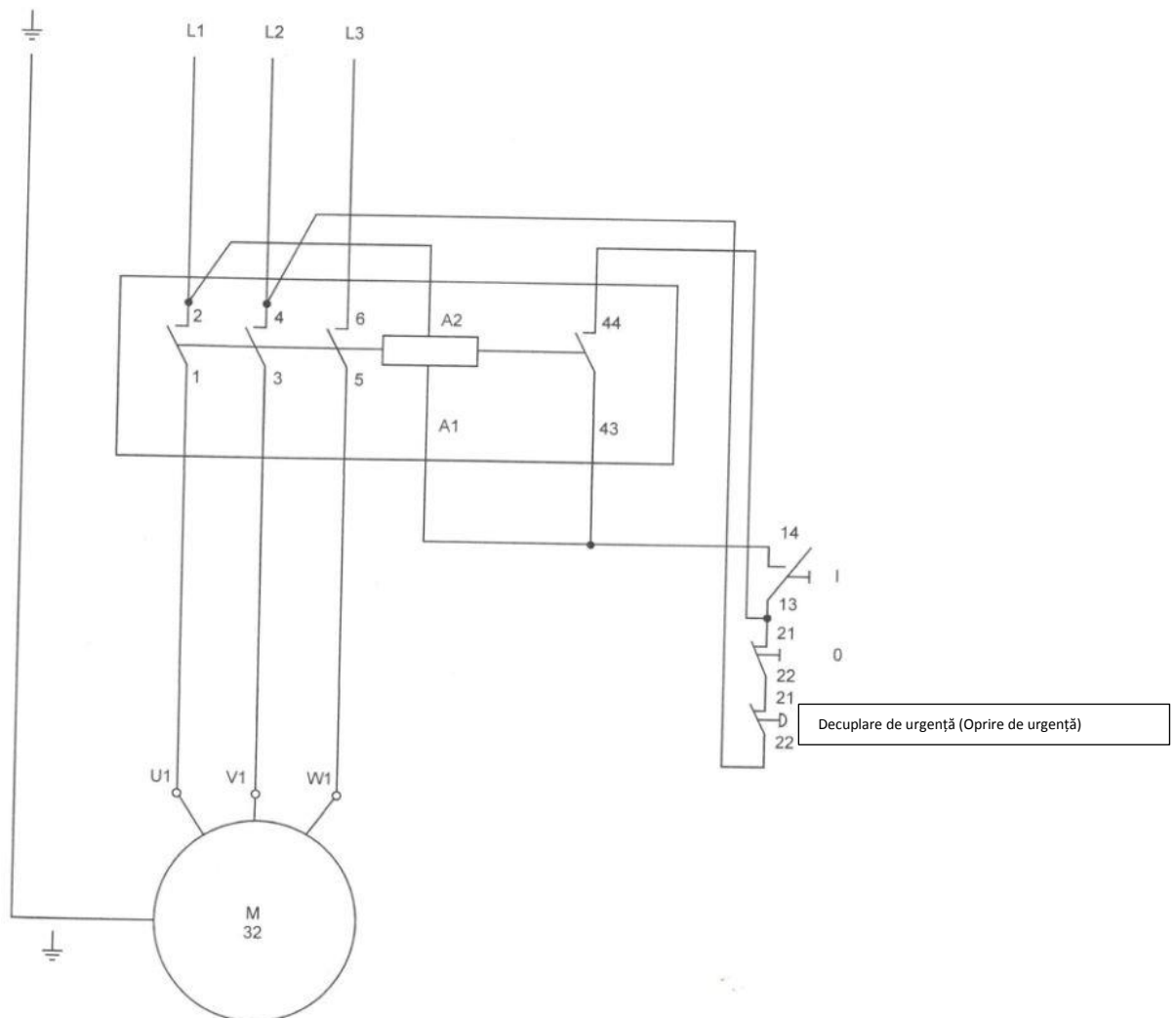
2. - schema de conectare a aparatului GYD 400E
